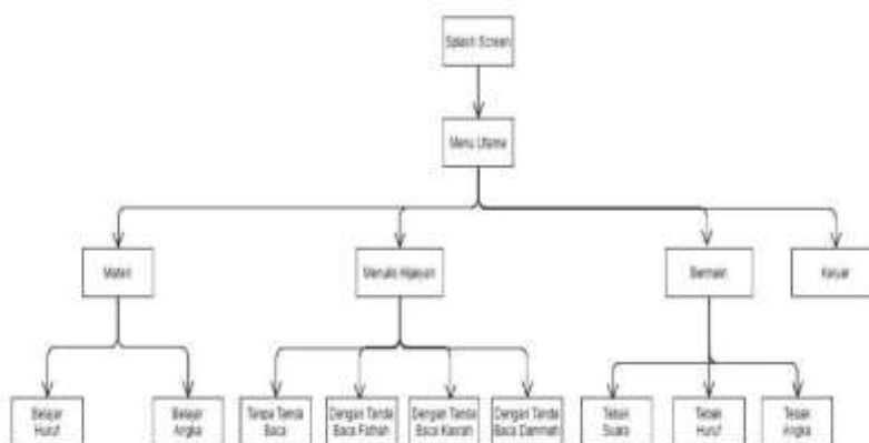
Gambar 24 Struktur Navigasi
