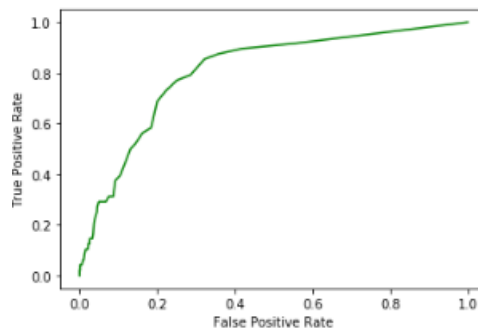
Gambar. 7. Grafik probabilitas model Random Forest dengan jumlah pohon 90.
