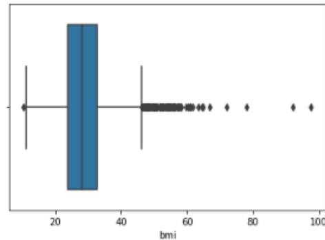
Gambar. 4. Dari gambar boxplot di atas diketahui bahwa atribut bmi mengandung data outlier .
