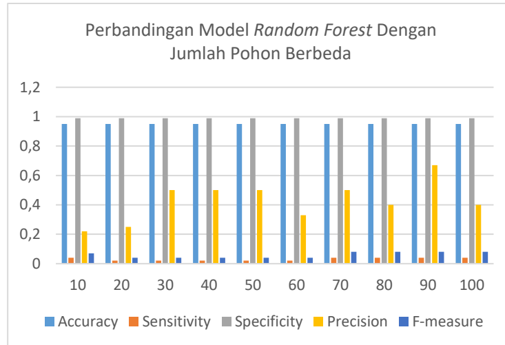
Gambar. 6. Bar chart model Random Forest dengan jumlah pohon berbeda. Warna biru muda mewakili accuracy , warna orange mewakili sensitivity , warna abu mewakili specificity , warna kuning mewakili precision , dan warna biru tua mewakili F-measure .
