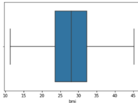
Gambar. 5. Setelah diperiksa kembali didapatkan bahwa atribut bmi telah bersih dari data outlier .
