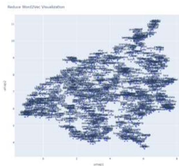
Gambar 3: Vektor space
